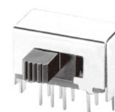
SK-23E01(2P3T)
